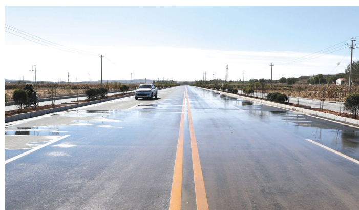
沁县208国道樊村段至南涅水石刻馆旅游公路路线走向由南向北,该线采用二级公路标准,设计速度60Km/h,路基宽度30m,行车道宽15.5m,非机动车道3.5m,人行道2m,绿化带1.75m,路缘带0.5m。总投资13358.7万元,目前主路段已完成油面铺装。秦超 牛佳丽摄影报道
